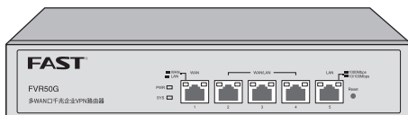
图1-1 FVR50G前面板示意图
